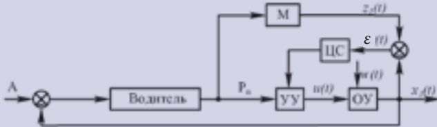
Рисунок 2. Структурная схема адаптивной системы тормозного управления с эталонной моделью
