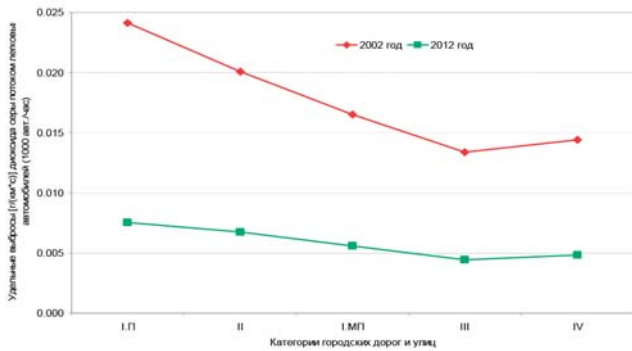
Рисунок 8. Изменение удельных выбросов диоксида серы [г/(км 3 )] для транспортного потока 1 000 ЛА/ч на городских дорогах и улицах различных категорий в 2002 и 2012 годах
