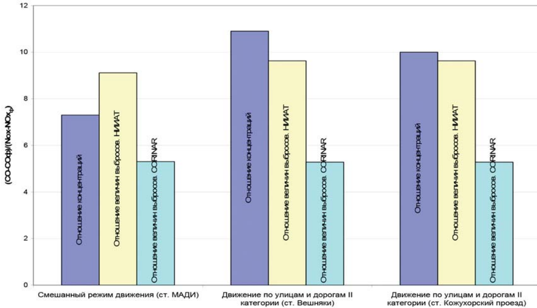
Рисунок 3. Отношение концентраций в воздухе на примагистральных территориях и расчётных величин выбросов CO/NO x
