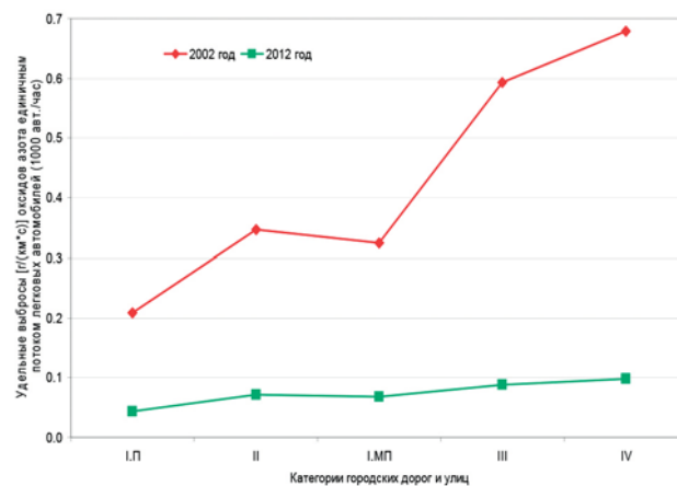
Рисунок 7. Изменение удельных выбросов оксидов азота [g/(км×с)] для транспортного потока 1 000 ЛА/ч на городских дорогах и улицах различных категорий в 2002 и 2012 годах
