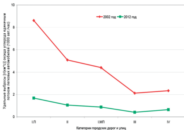
Рисунок 6. Изменение удельных выбросов монооксида углерода [g/(км×с)] для транспортного потока 1 000 ЛА/ч на городских дорогах и улицах различных категорий в 2002 и 2012 годах
