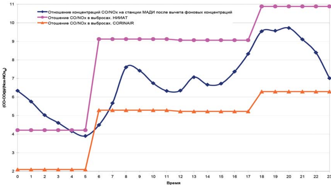
Рисунок 4. Внутрисуточный ход отношений величин выбросов и концентраций CO и NO x в воздухе
